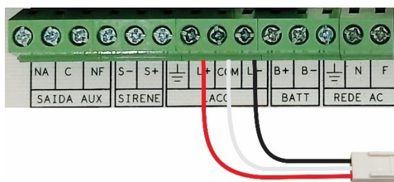
Figura 4. 12: Conexão chicote de programação de sensores na central.
