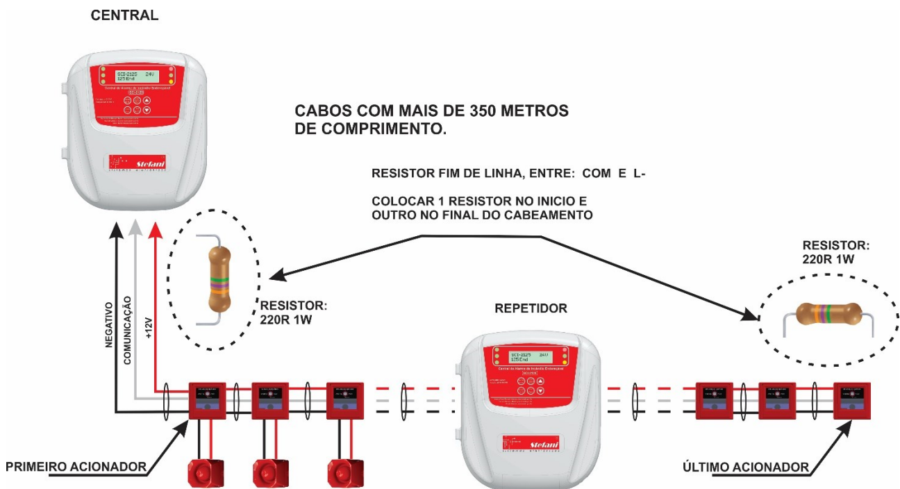
Figura 5. 7: Esquema de ligação com repetidor na metade do cabeamento.
