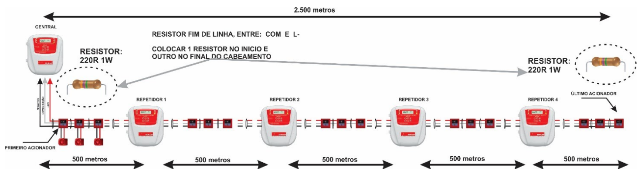
Figura 5. 9: Esquema de ligação para cabeamento com 1.600 metros.
