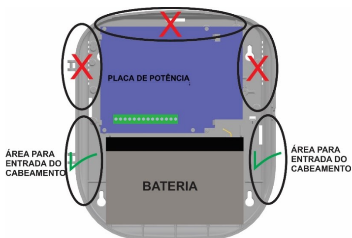
Figura 5. 1: Áreas corretas e incorretas para entrada do cabeamento.
