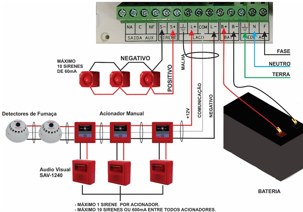
Figura 5. 5: Esquema de ligação do sistema.
