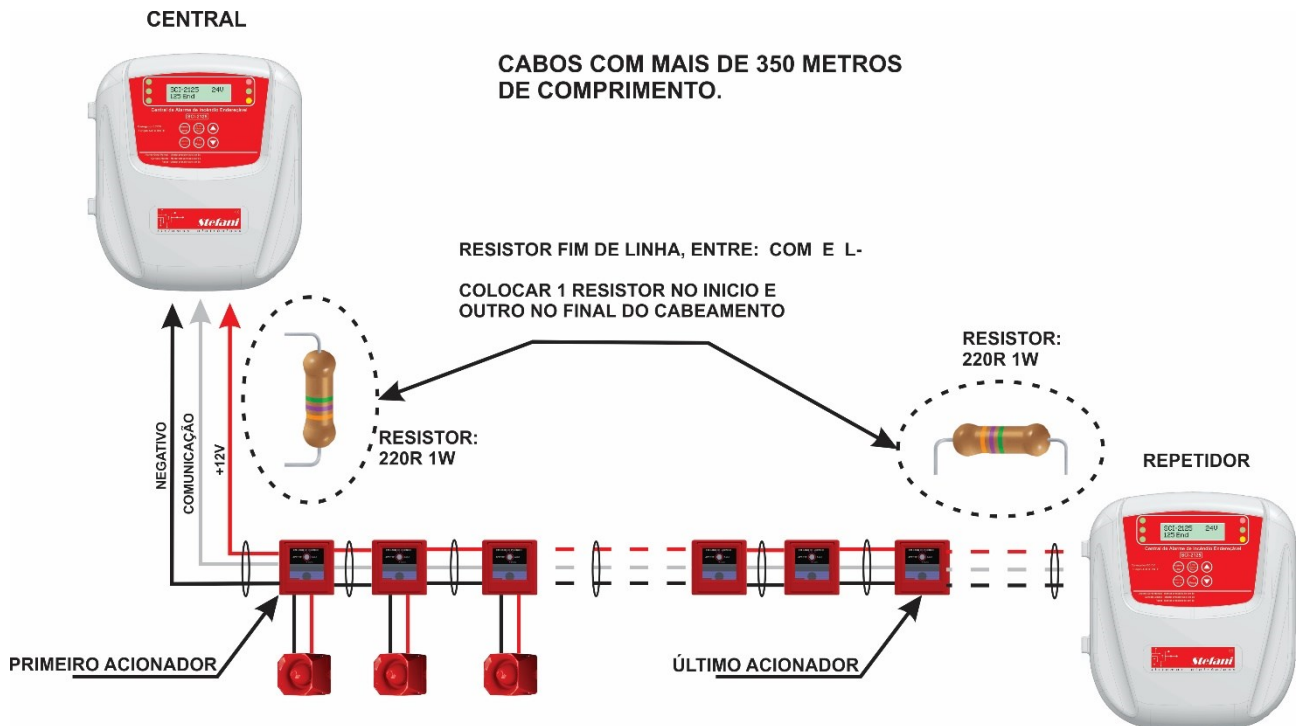
Figura 5. 8: Esquema de ligação com repetidor no final do cabeamento.
