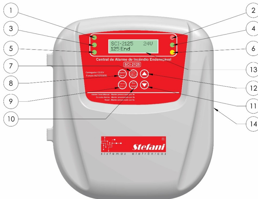
Figura 2. 1: Legenda de funções da Central
