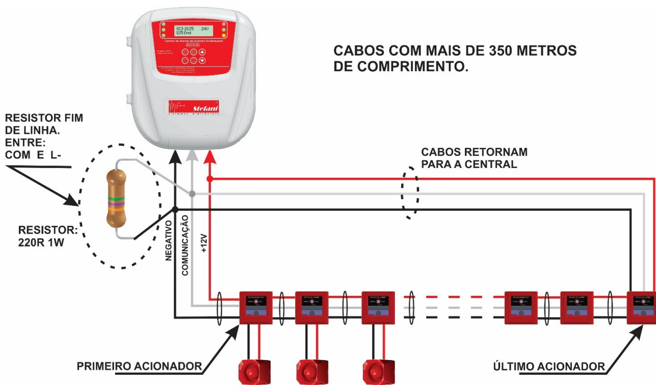
Figura 5. 6: Configuração em LOOP.
