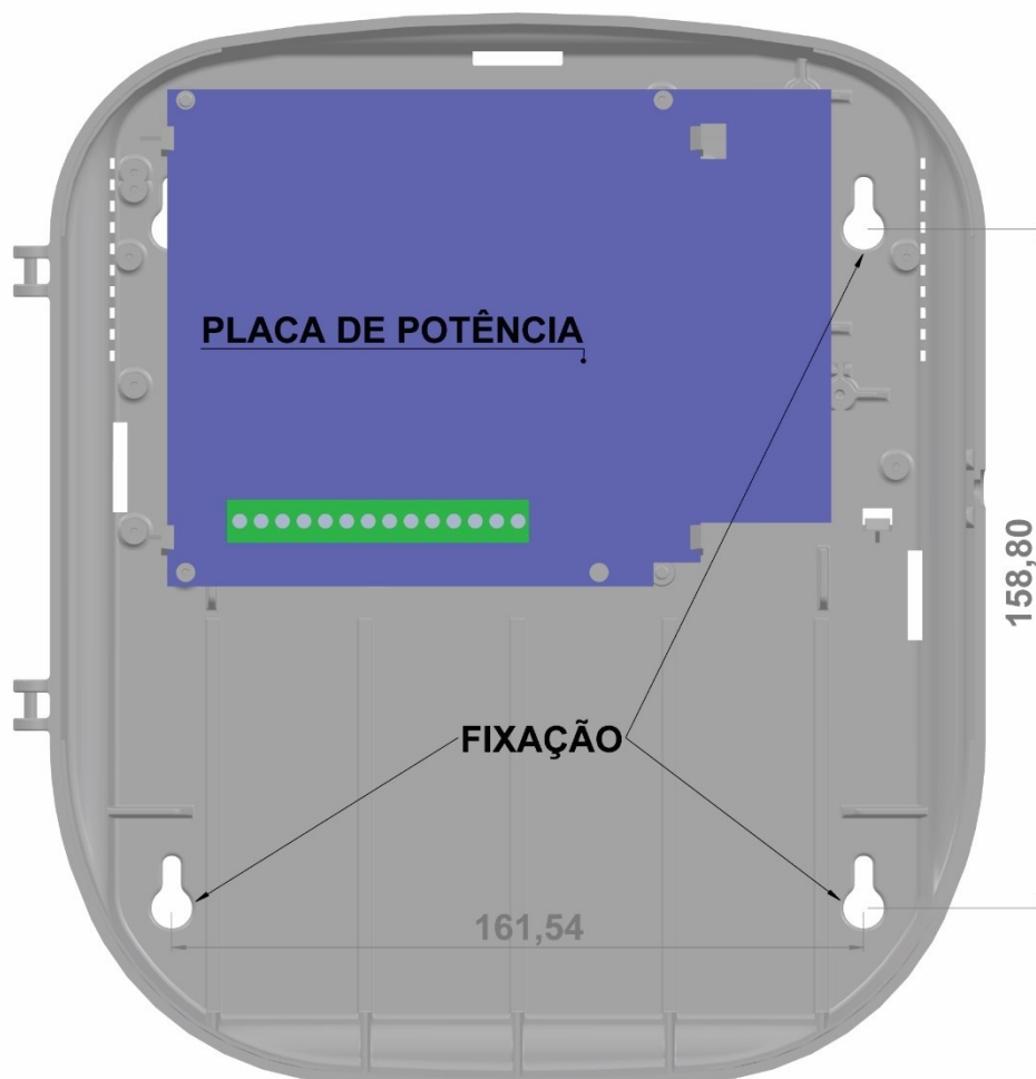
Figura 5. 2: Locais destinados para fixação da central.
