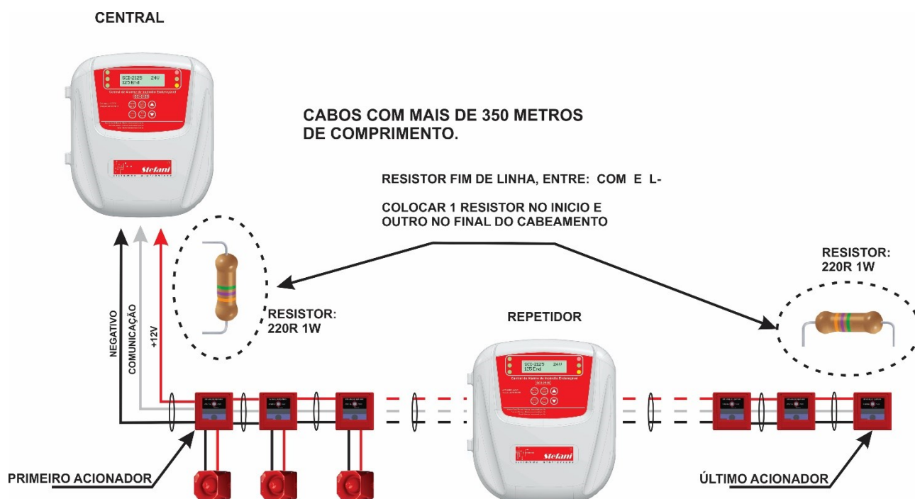
Figura 5. 9: Esquema de ligação com repetidor na metade do cabeamento.
