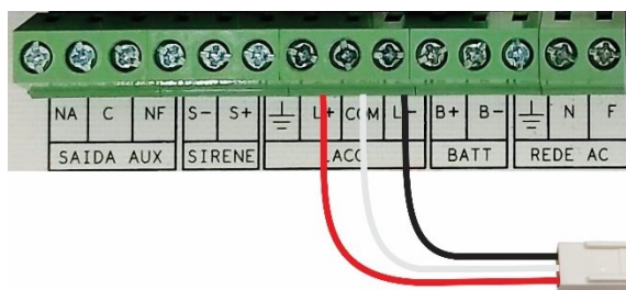
Figura 4. 10: Conexão chicote de programação de sensores na central.
