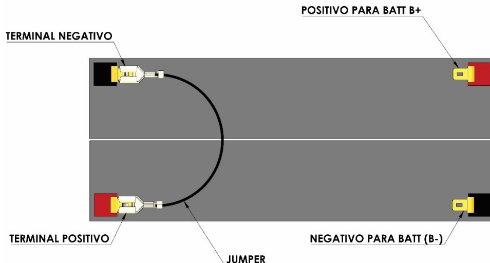
Figura 5. 6: Montagem das baterias.
