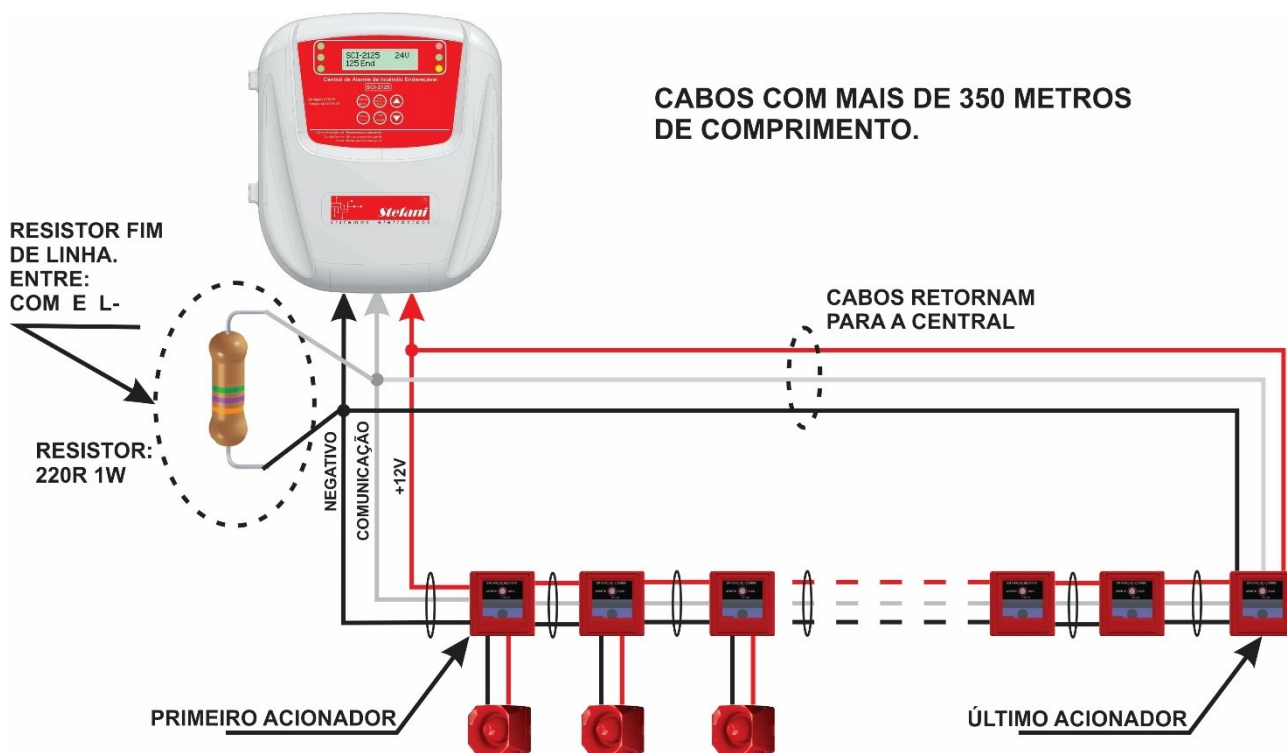
Figura 5. 8: Configuração em LOOP.
