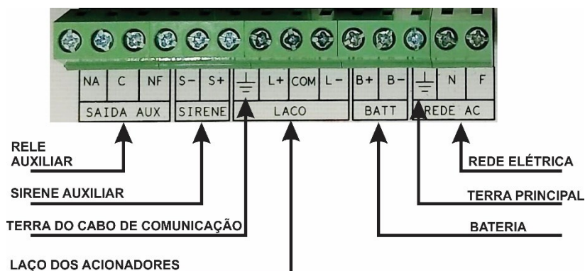
Figura 5. 3: Legenda do conector de ligação.
