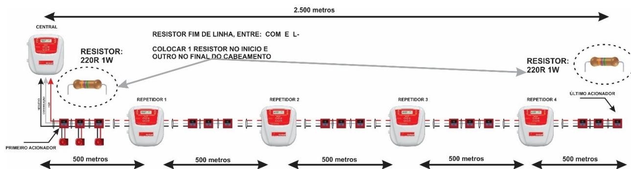
Figura 5. 11: Esquema de ligação para cabeamento com 2.500 metros.
