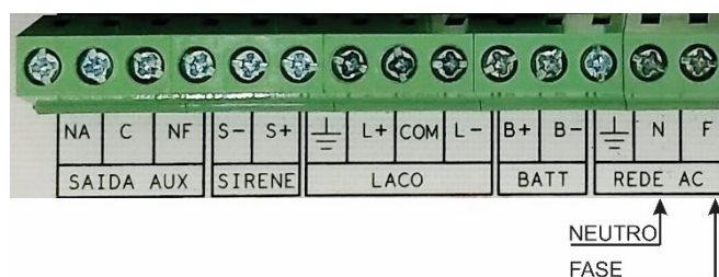
Figura 4. 1: Ligação rede elétrica.
