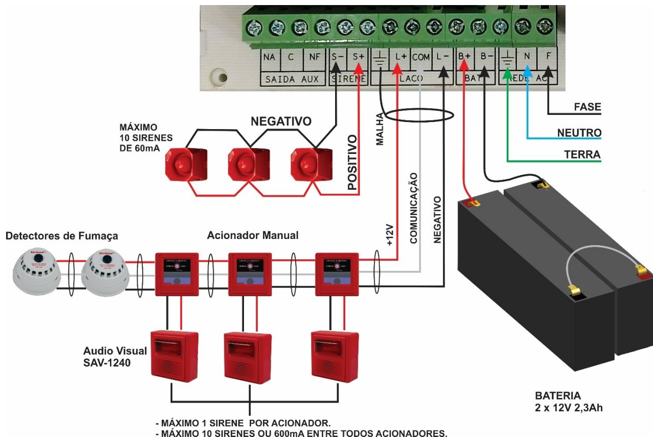
Figura 5. 5: Esquema de ligação do sistema.
