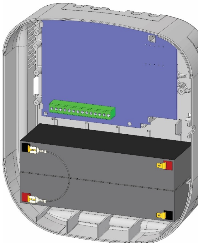
Figura 5. 7: Acomodação das baterias dentro do gabinete.
