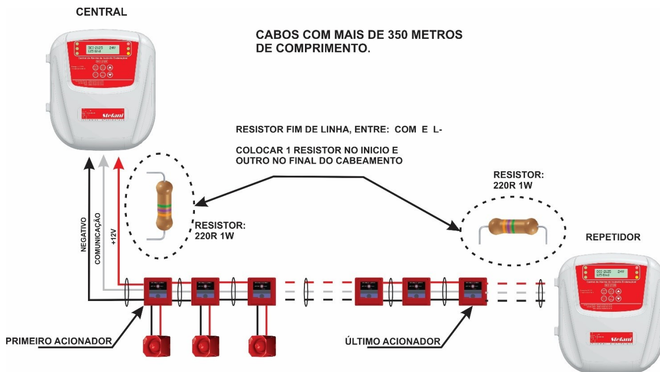
Figura 5. 10: Esquema de ligação com repetidor no final do cabeamento.
