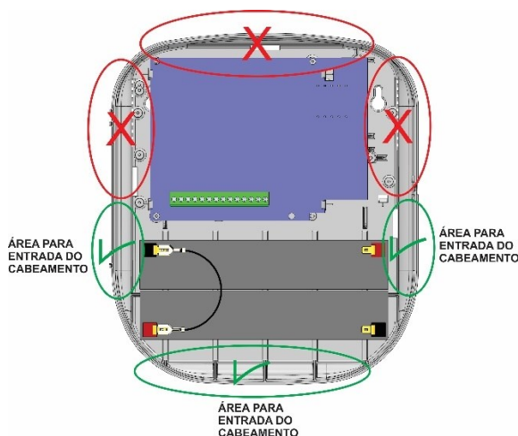
Figura 5. 1: Áreas corretas (✓) e incorretas (X) para entrada do cabeamento.
